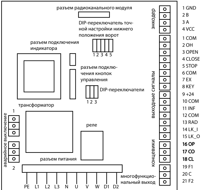
Рис. 12 Расположение элементов на плате GYK-92SY
