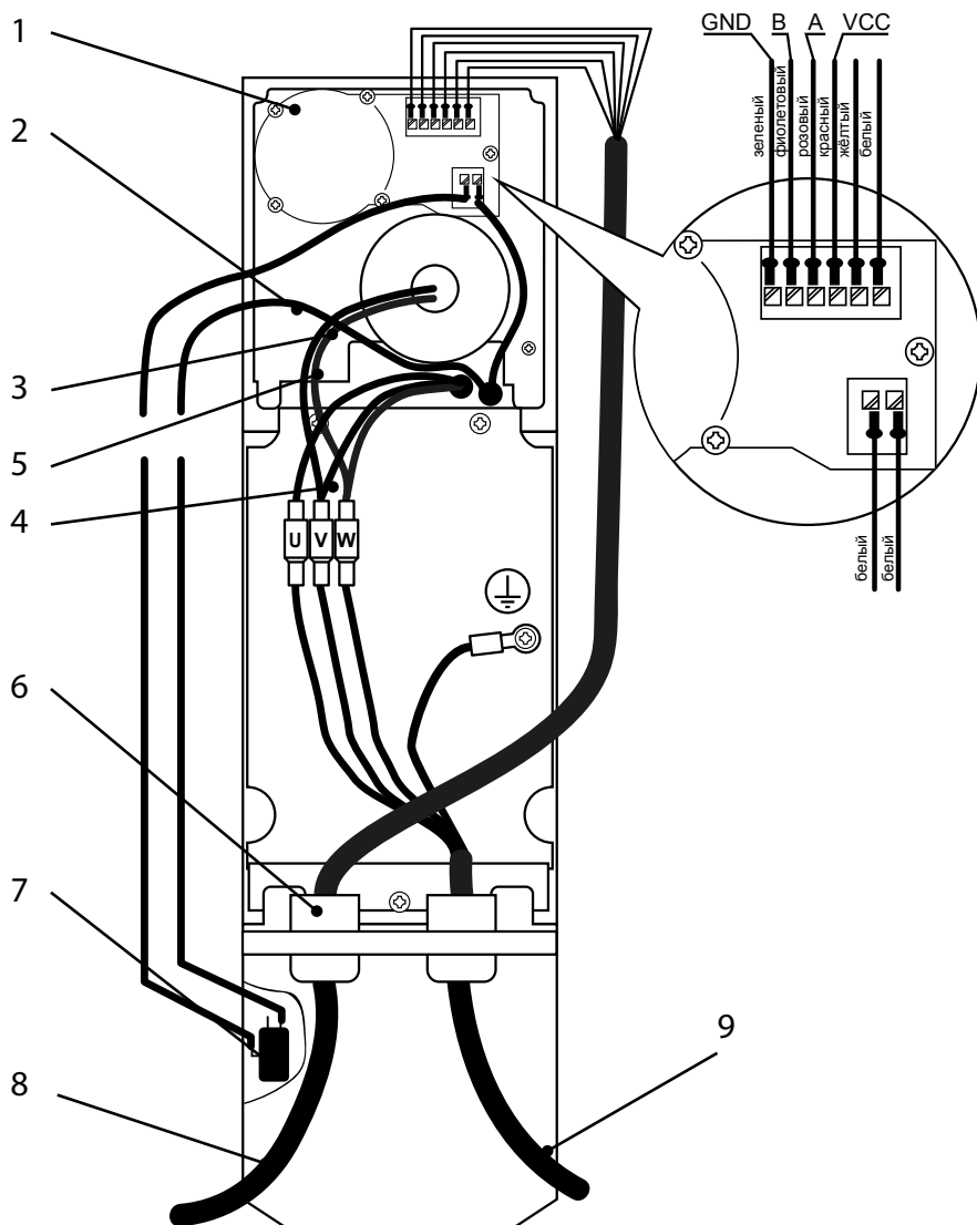
Рис. 9 Схема подключения привода
