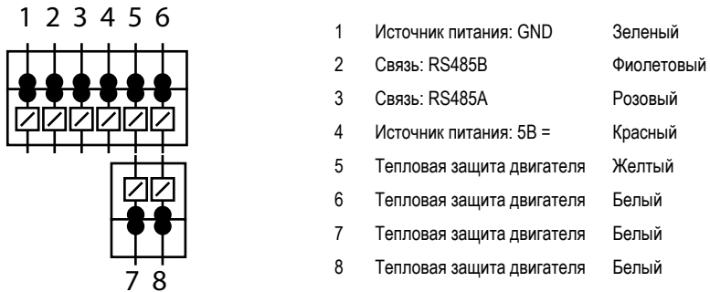
Рис. 10 Распайка клеммной колодки
