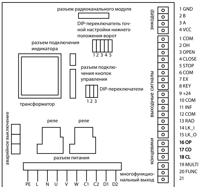
Рис. 11 Расположение элементов на плате GYK-92Y
