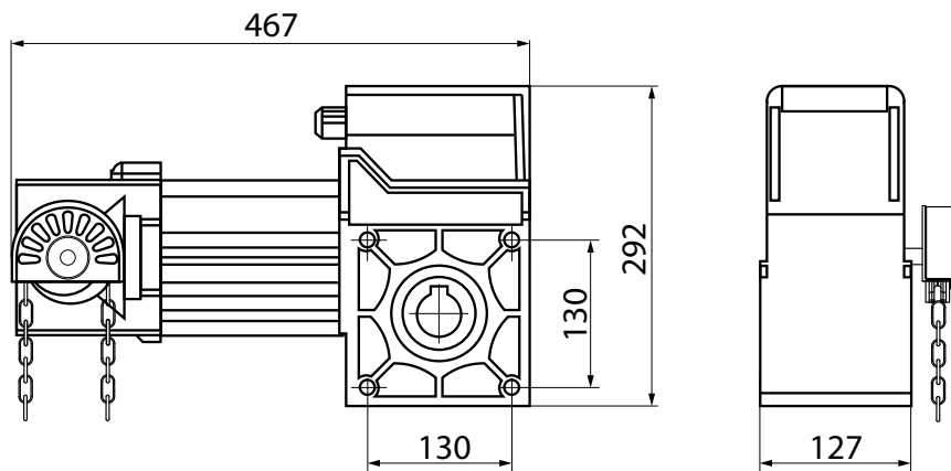
Рис. 3 Габариты привода RSI200-2EL
