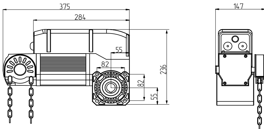
Рис. 2 Габариты приводов RSI50-2EL, RSI70-2EL, RSI100-2EL, RSI150-2EL
