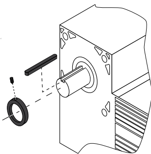
Рис. 5 Схема установки шпонки и втулки на вал секционных ворот
