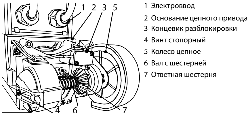
Рис. 7 Устройство ручного цепного привода (крышка снята)
