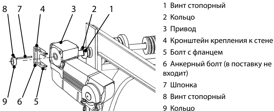
Рис. 4 Схема установки привода на вал секционных ворот
