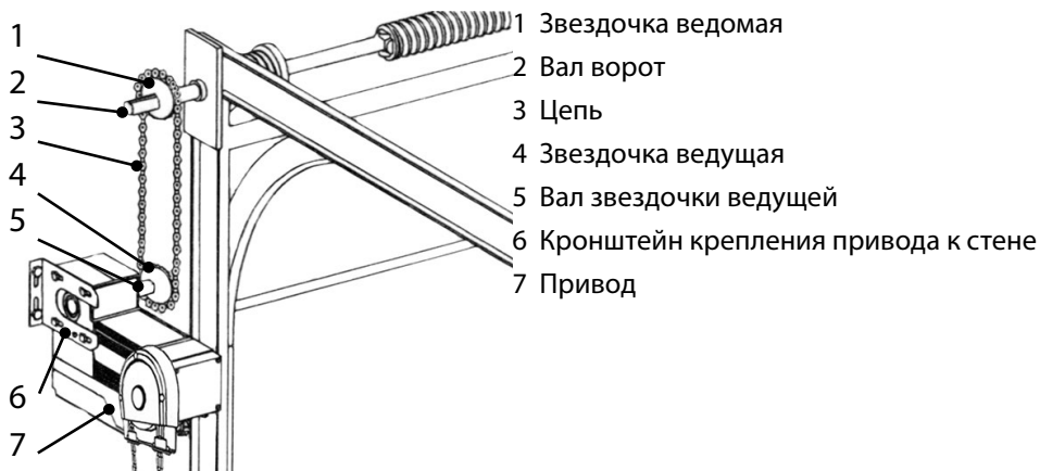
Рис. 6 Схема установки привода на вал секционных ворот
